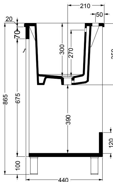
SEZIONE A-A'
