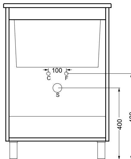
VISTA FRONTALE SENZA ANTE
