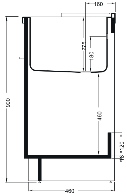
SEZIONE A-A
