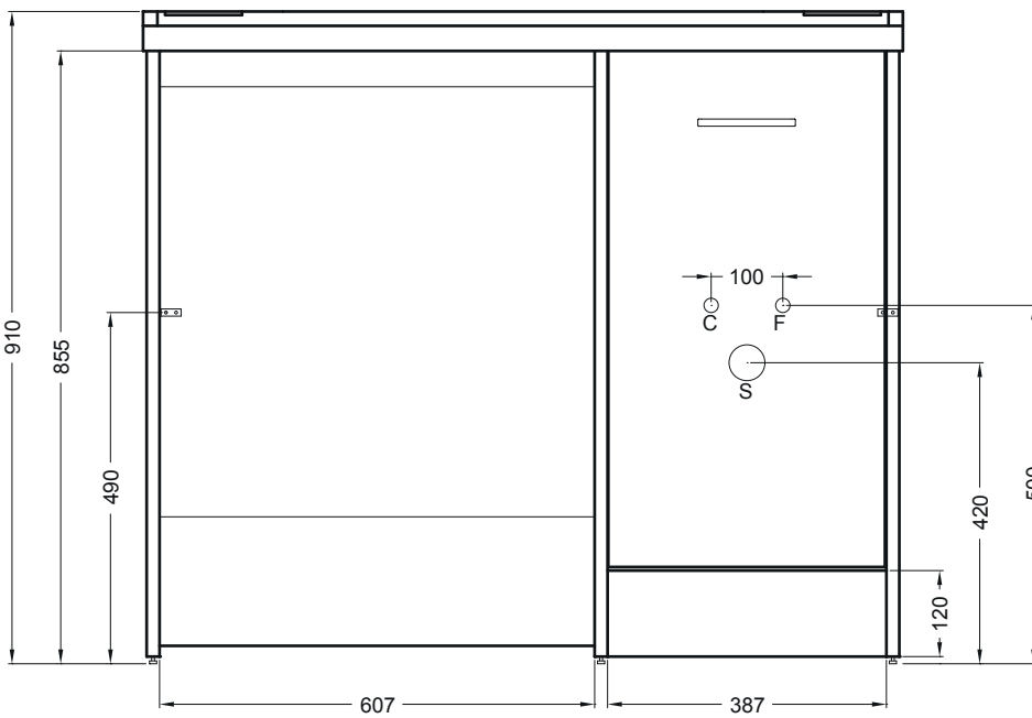
VISTA FRONTALE
