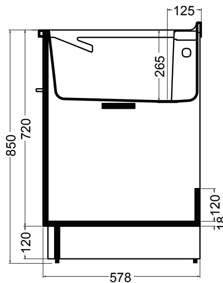
SEZIONE A-A'
