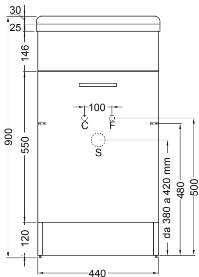
VISTA FRONTALE
