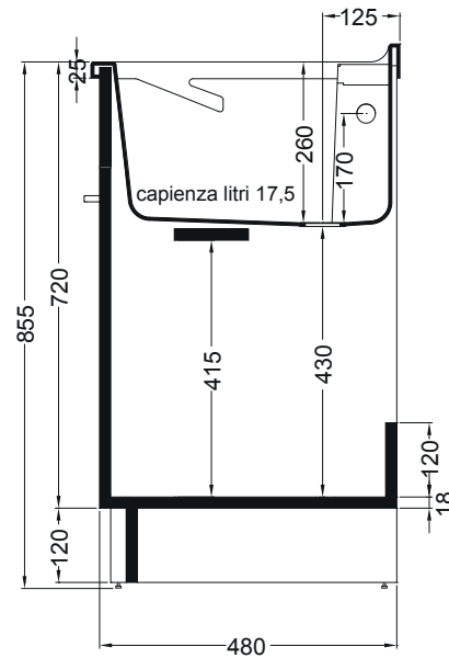
SEZIONE A-A'
