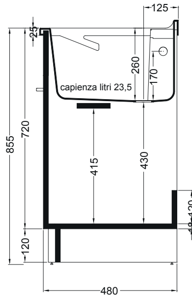
SEZIONE A-A'
