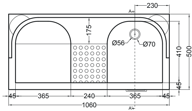
PIANTA
