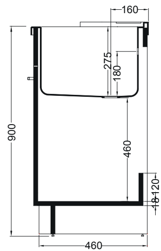
SEZIONE A-A'
