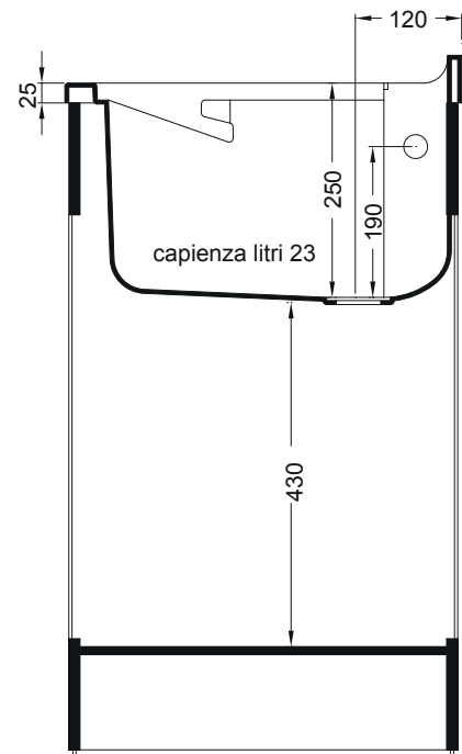
SEZIONE A-A
