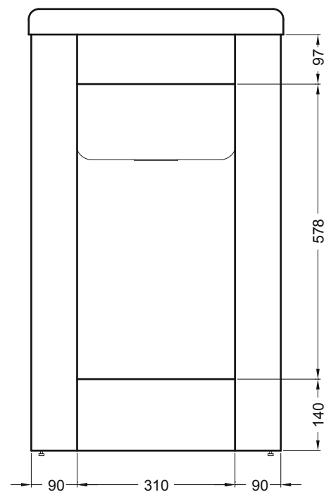
VISTA POSTERIORE
