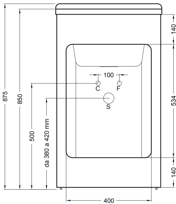
VISTA FRONTALE
