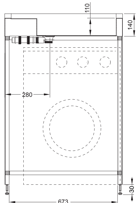
SEZIONE A-A
