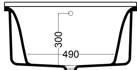
SEZIONE B-B
