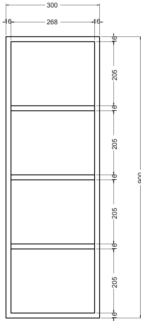
VISTA FRONTALE
