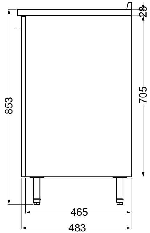
VISTA LATERALE
