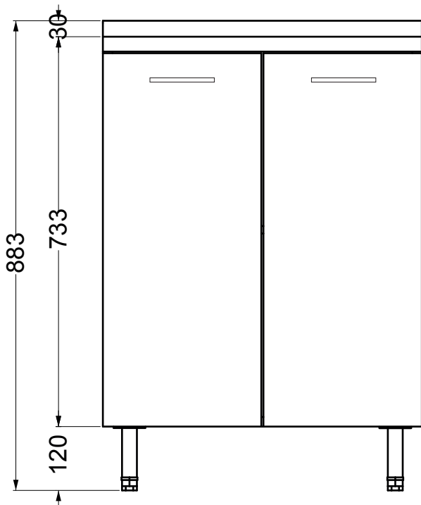
VISTA FRONTALE
