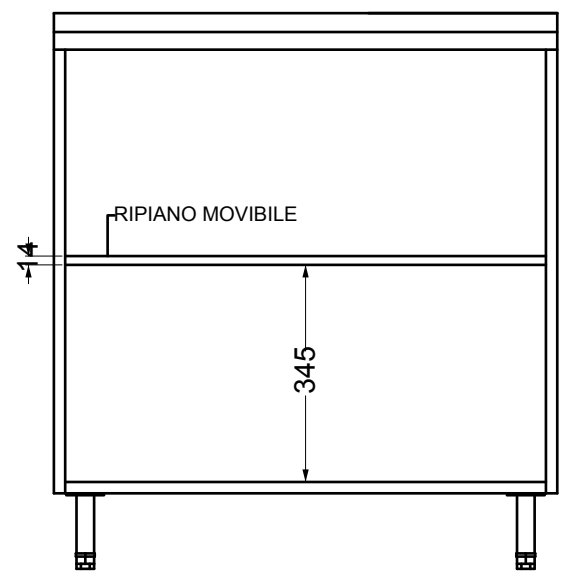
VISTA FRONTALE SENZA ANTE
