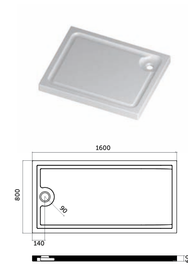
Piatto doccia 160x80 Shower-tray 160x80 antiscivolo/ anti-slip COD. PD16080601
