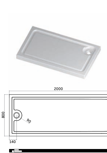
Piatto doccia 200x80 Shower-tray 200x80 antiscivolo/ anti-slip COD. PD20080601
