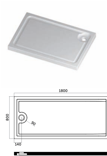
Piatto doccia 180x80 Shower-tray 180x80 antiscivolo/ anti-slip COD. PD18080601
